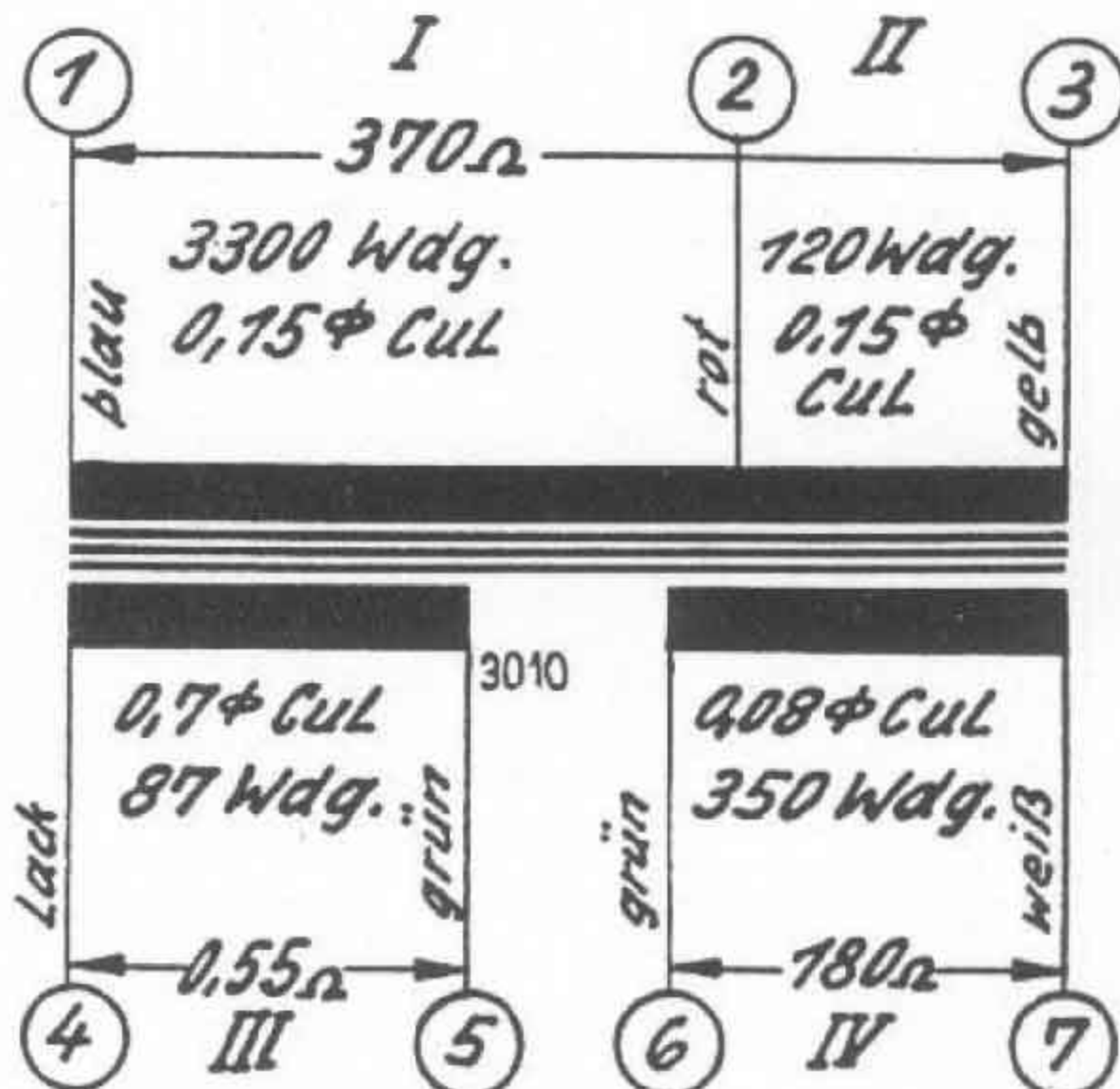
Übertrager BV 60/55
