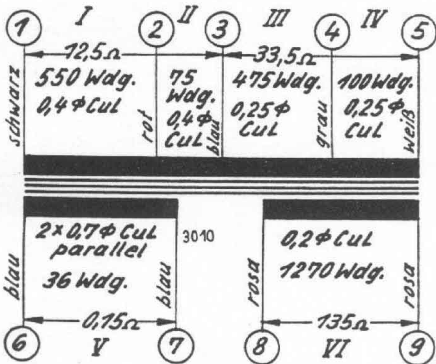
Netztransformator BV 84/19
